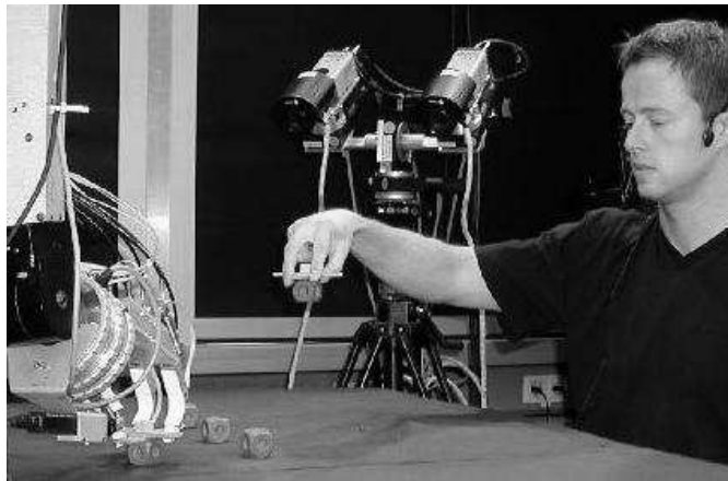
Abbildung 7: Angestrebtes Imitationsszenario und nach dem Vorbild menschlicher Griffposturen eingestellte, "wirkungsäquivalente" Posturen der Roboterhand des GRAVIS-Systems.
